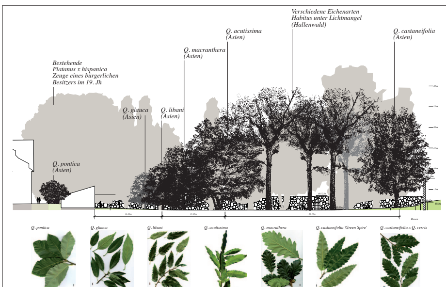
Schnittansicht Arboretum
