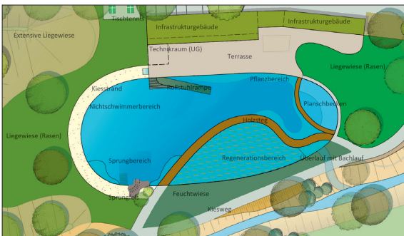
Ausschnitt aus dem Konzeptplan mit Fokus auf den Badesee
