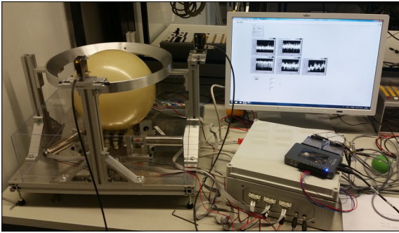
Prototyp optischer CO 2 -Sensor co 2
